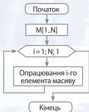
Опрацювання елементів одновимірного масиву M[1..N]
